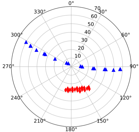
(b) PROBA-V
