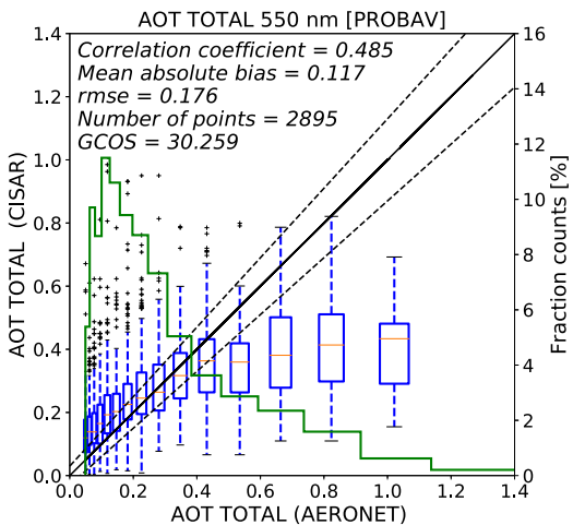
(b) PROBA-V
